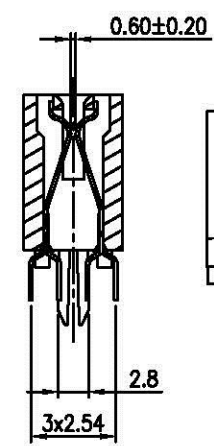
METAL CLIP
